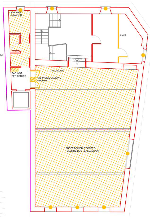
PLANTA SEGONA
