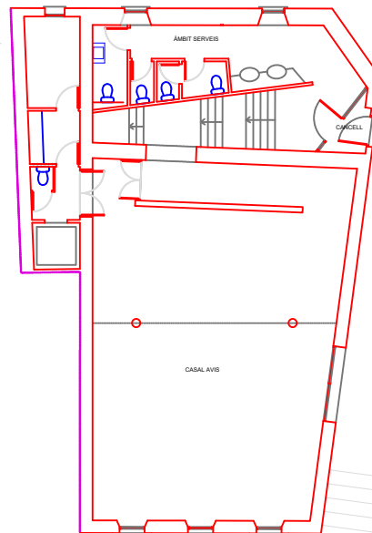
PLANTA PRIMERA
