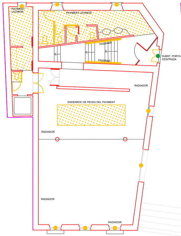
PLANTA PRIMERA
