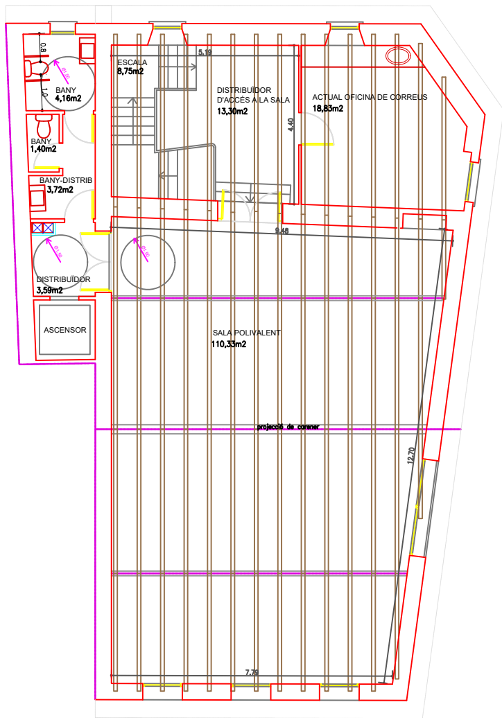
PLANTA SEGONA
